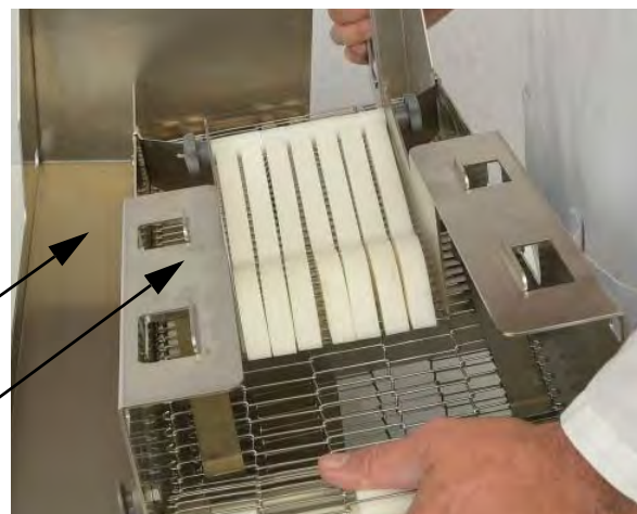
Assemblage de convoyeur de panure
